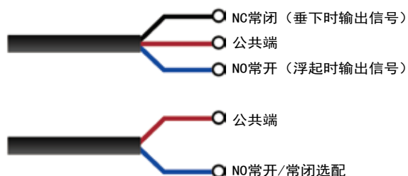
排 线 图
