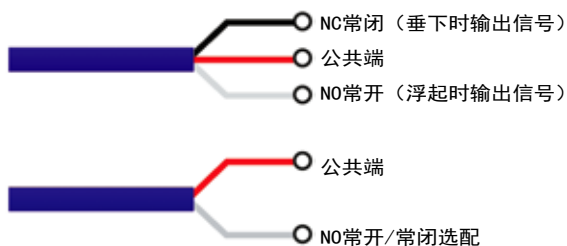
排 线 图
