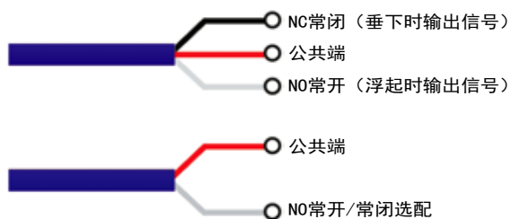
排 线 图
