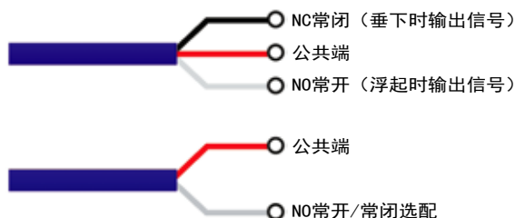
排 线 图
