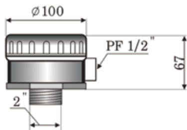
产 品 图 尺 寸
