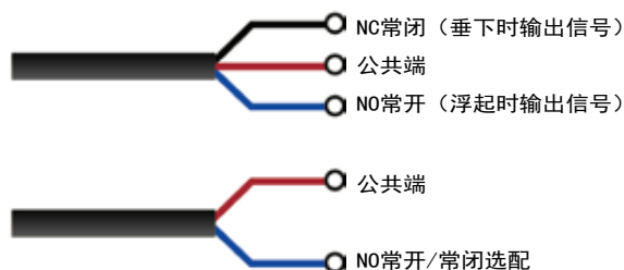
排 线 图
