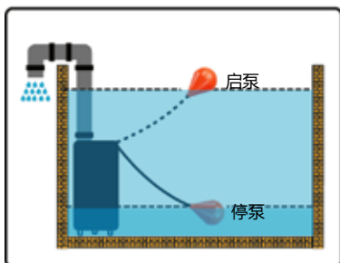
安 装 方 法
